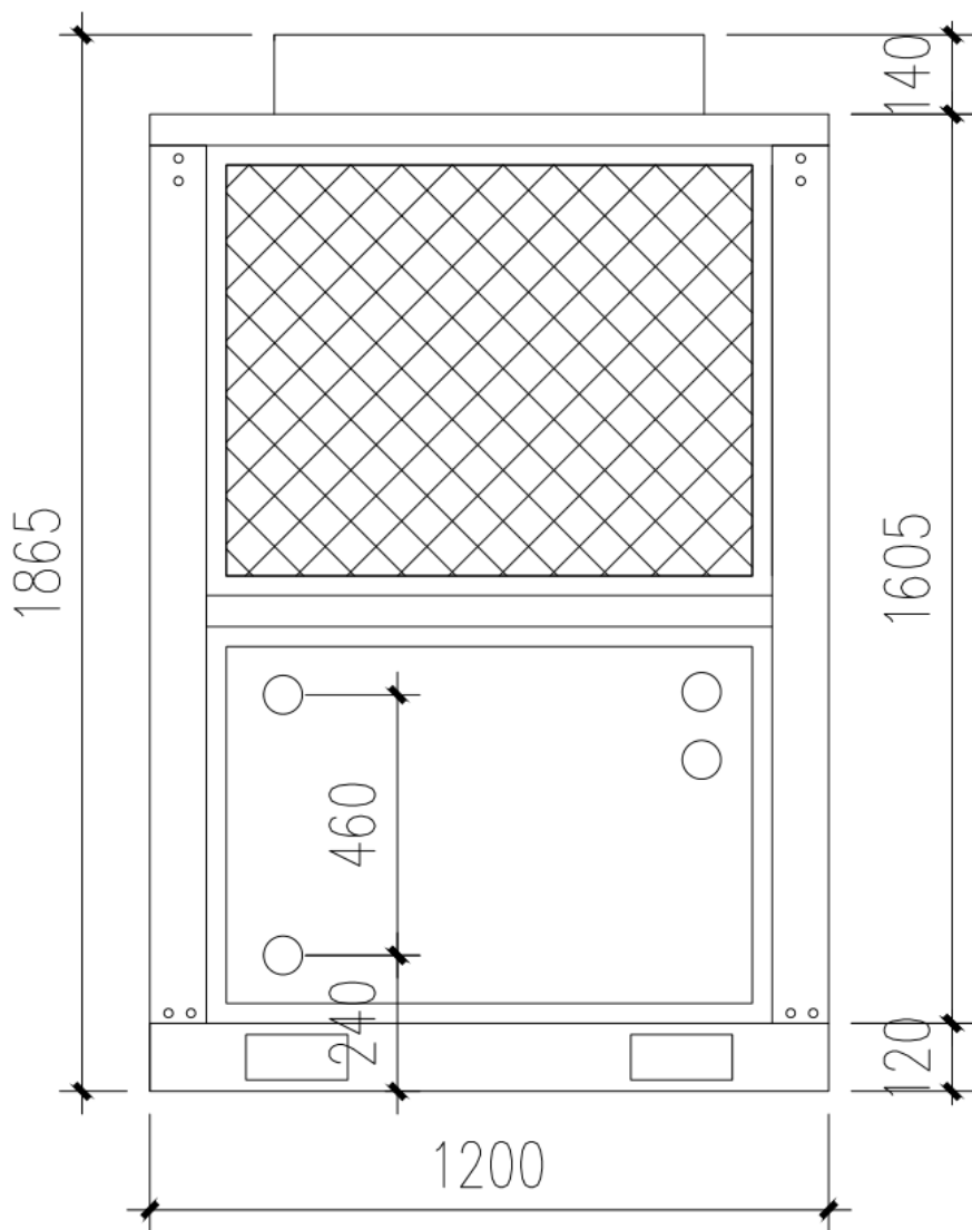
b、机组宽*高及进出水口尺寸图
