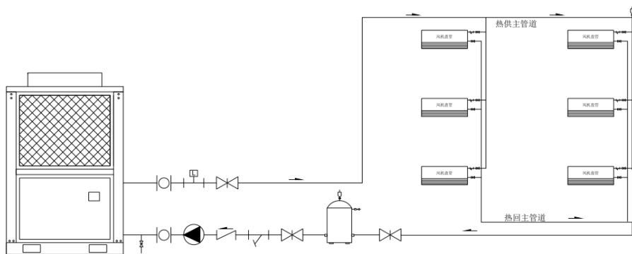
注：上图为风机盘管冷暖闭式循环系统安装图。
