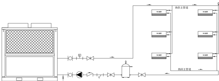
注：上图为风机盘管冷暖闭式循环系统安装图。
