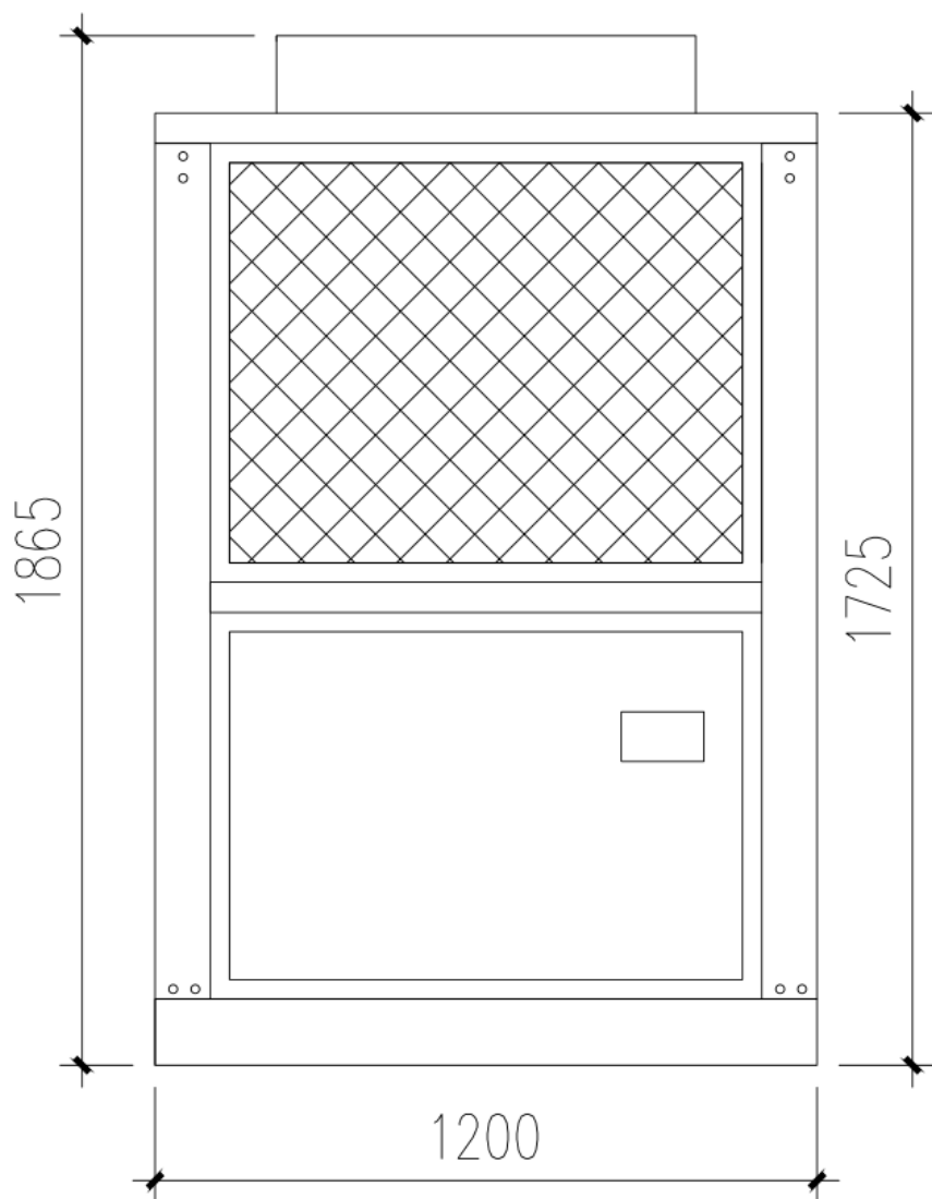
b、机组宽*高外形尺寸图
